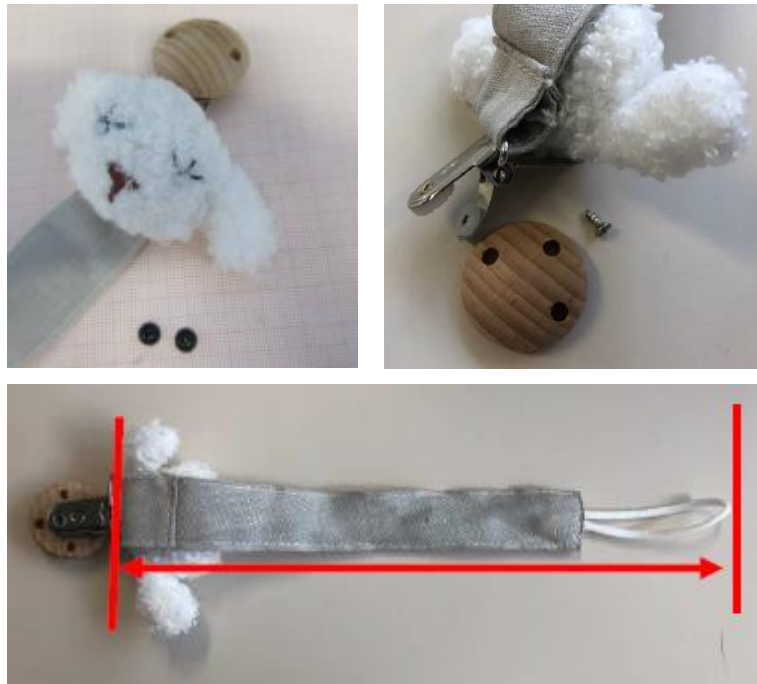
Figure 2. Illustration de non-conformités à la norme EN 12586
